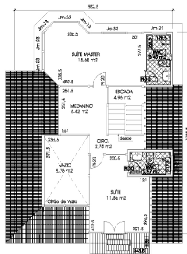
PLANTA PAV SUPERIOR
